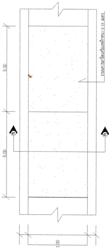
แบบถาดนคอนกรีตเสริมเหล็ก
