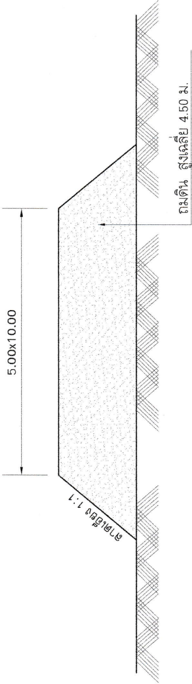
รูปตัดคั่นคลอง จุดที่ 3
