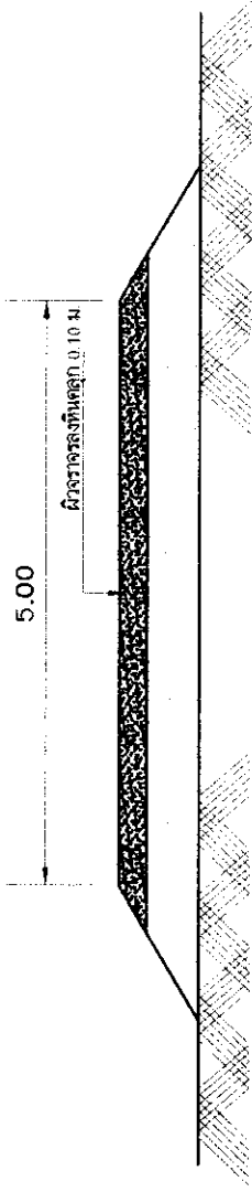
รูปตัดถนน
