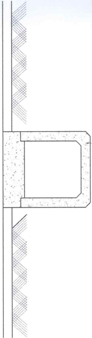
ร่างระบายนํ้า คสล. สำร็จรูป ขนาด 0.30 x 1.00 ม.
